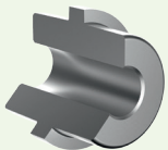
Gleitlager G Plain bearing G 滑轴 G
